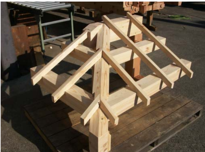
隅木レベルを下げて垂木を隅木の上端で納める方法です。
